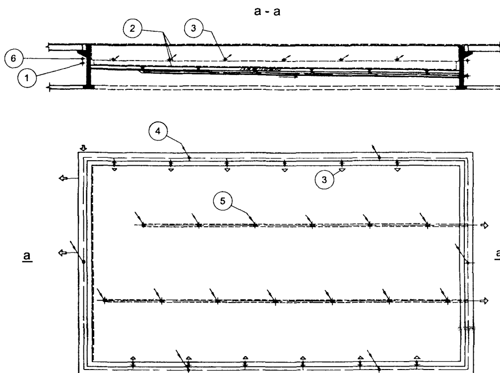
А. Бассейн 25×13,5 м
