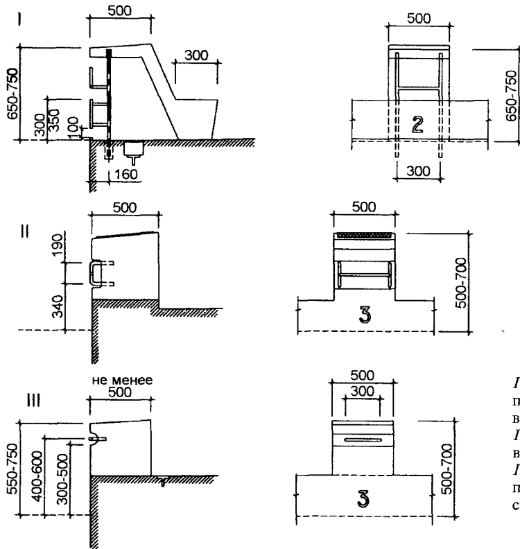
Схемы лестниц для выхода из ванны
