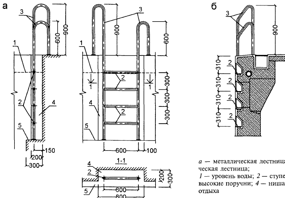
Схемы лестниц для выхода из ванны
